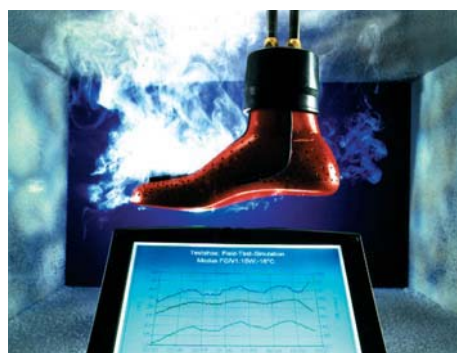
Cyborg – simulace různých klimatických podmínek pro testování prodyšnosti obuvi.
